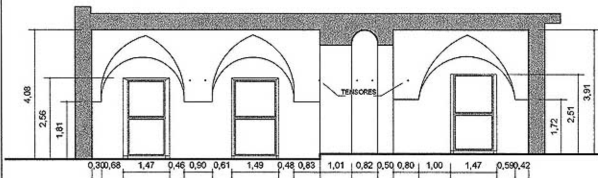
CORTE A-A
