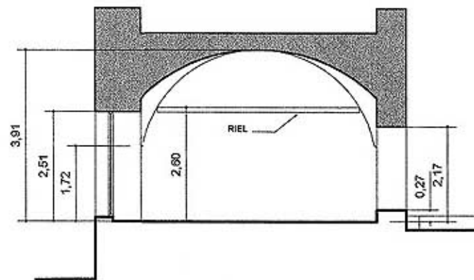
CORTE D-D
