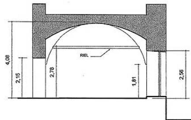
CORTE C-C
