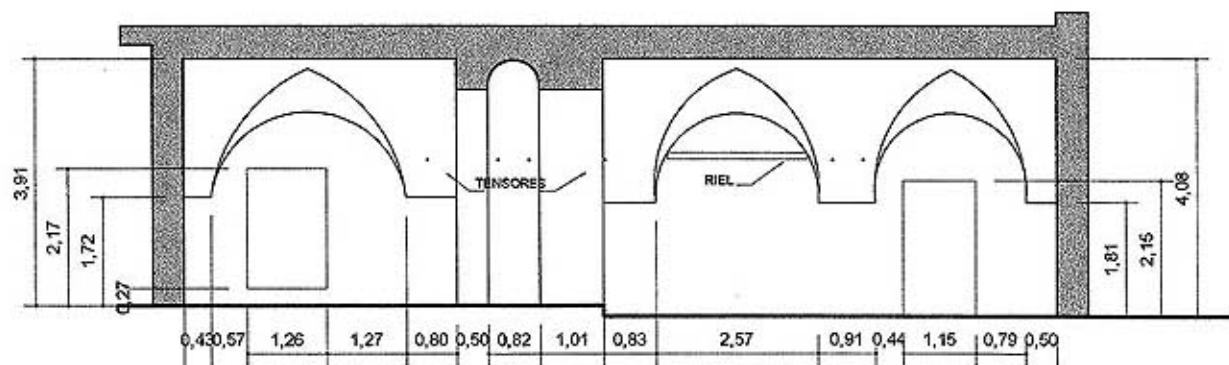
CORTE B-B
