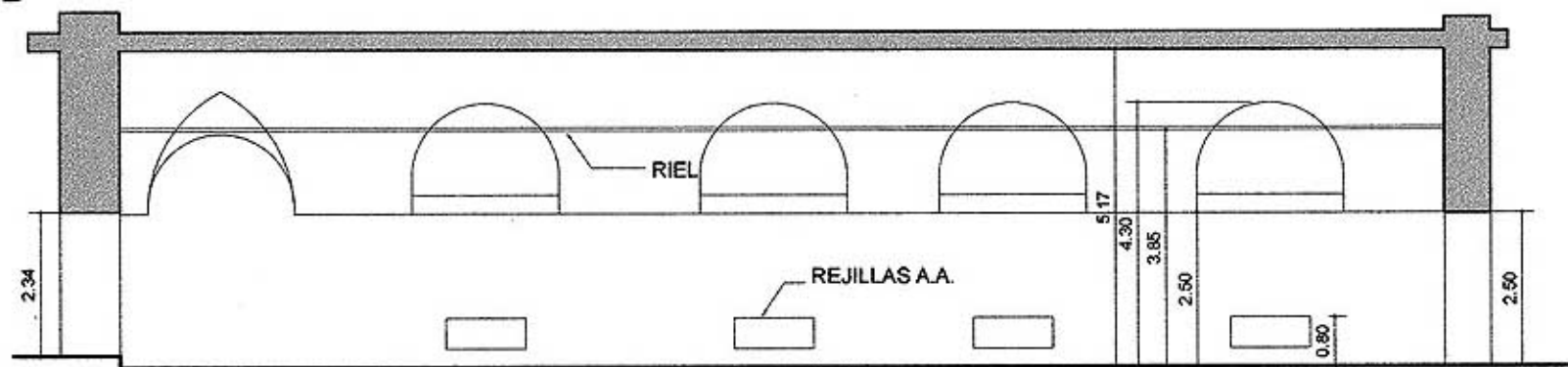
CORTE D-D
