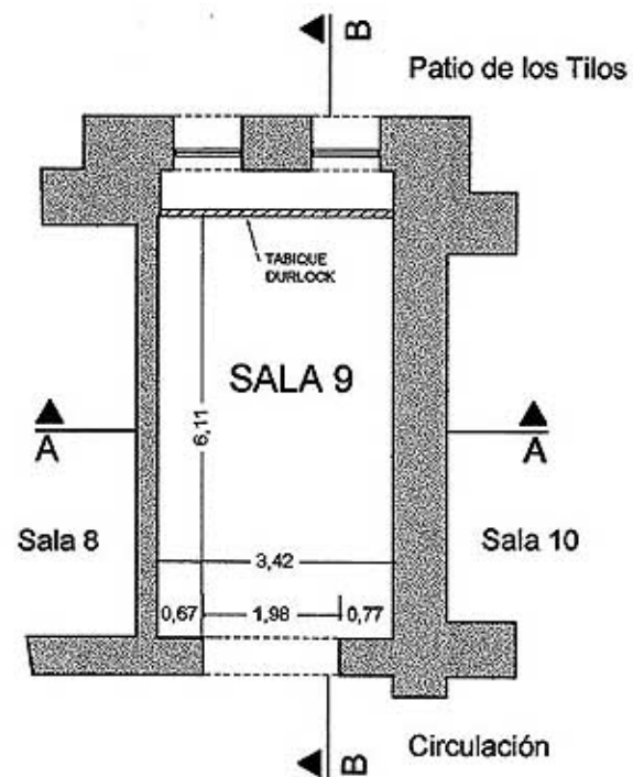
PLANTA
