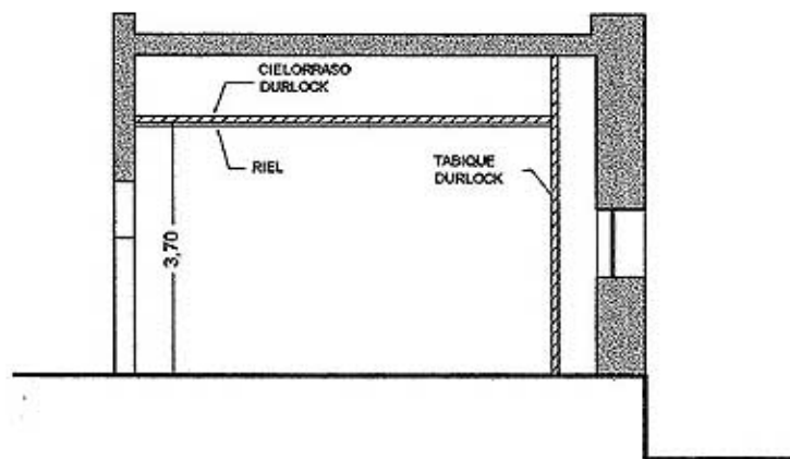
CORTE B-B
